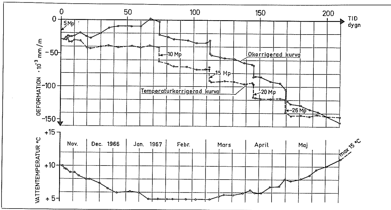
Fig 1. Påldel 1:s deformation med tiden vid stegvis ökande last samt kylvattnets temperaturvariation
